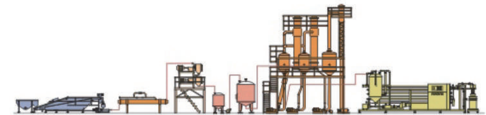
番茄酱流程示意图
